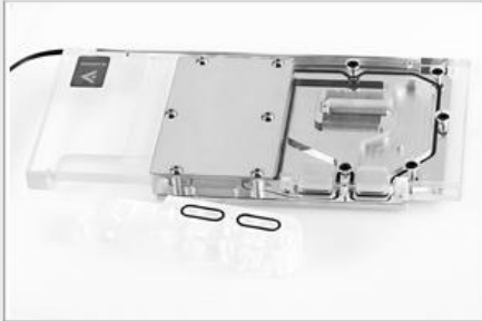
2. 将胶圈压入桥头胶圈槽内 (轻轻拽一下会更方便安装)
