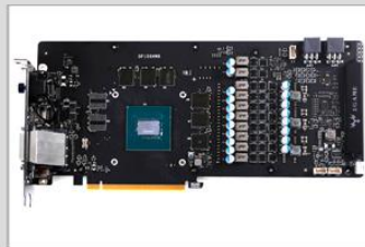
10. 清理并重新涂抹硅脂
